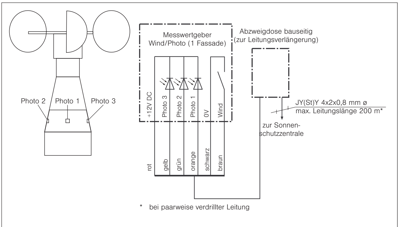
Abb. 3 Anschlussplan
